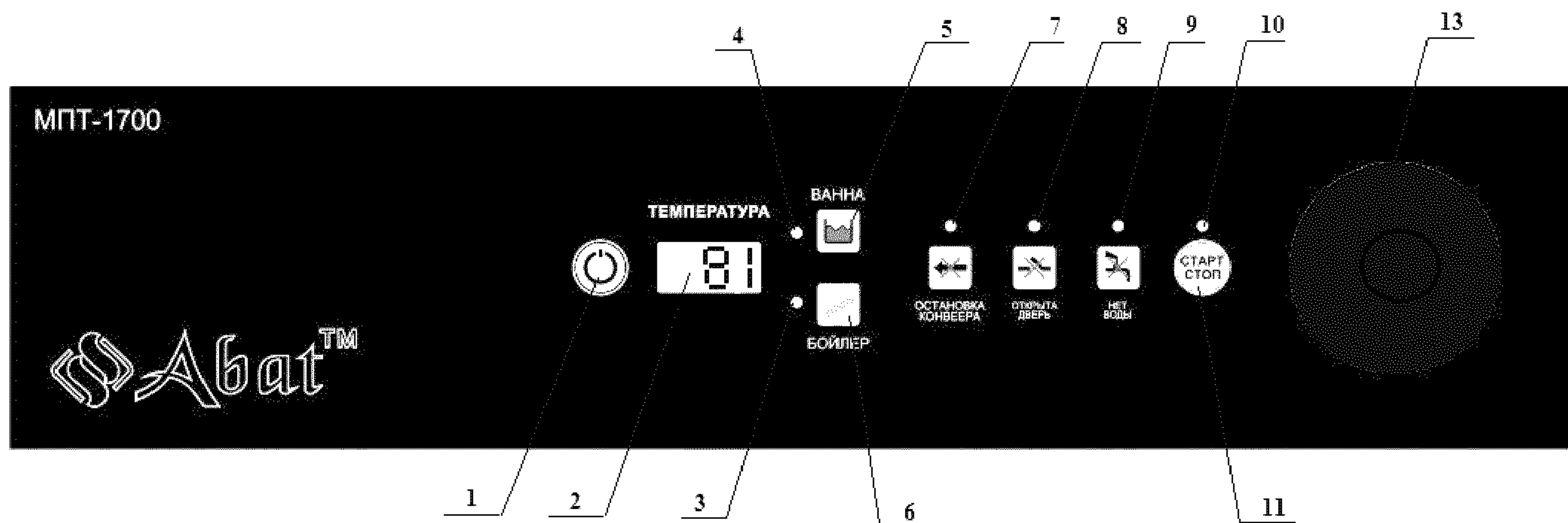
Рис. 2. Панель управления
